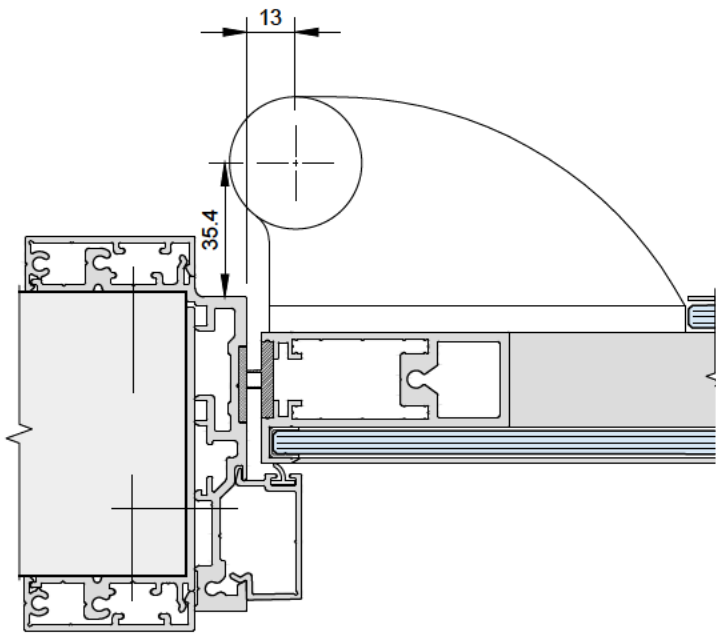
01 XP DOOR FRAME Scale: 1:2
