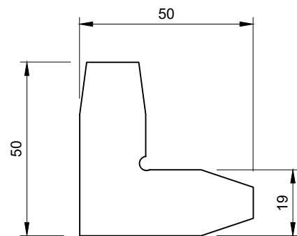
90° DOOR FRAME CLEAT S9DCLEAT90
