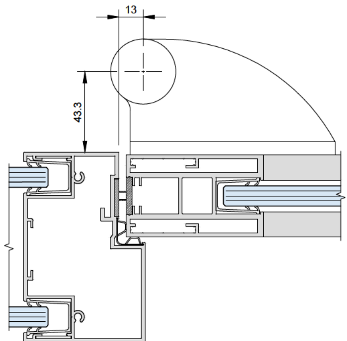
04 SYSTEM 9000 DG DOOR FRAME Scale: 1:2
