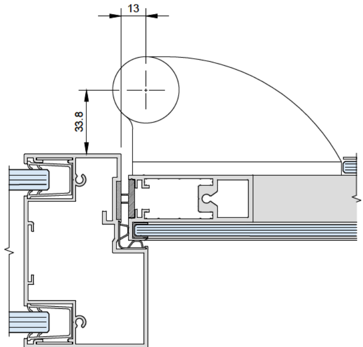
04 SYSTEM 9000 DG DOOR FRAME Scale: 1:2
