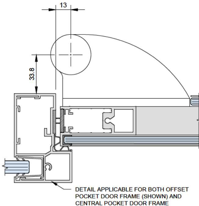
03 SYSTEM 9000 SG DOOR FRAME Scale: 1:2
